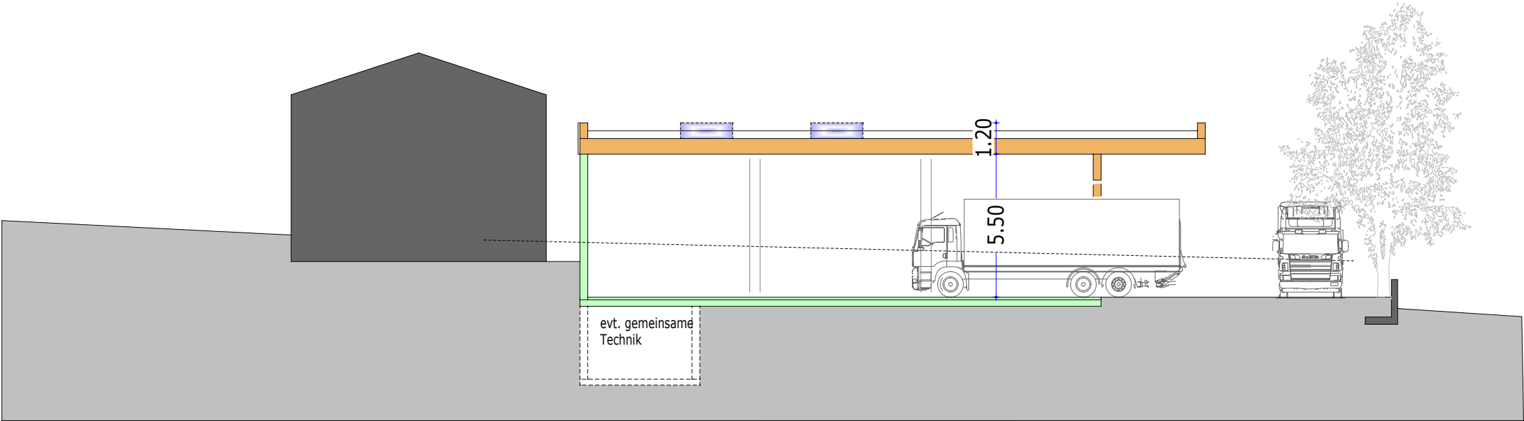
SCHNITT M: 1/250
