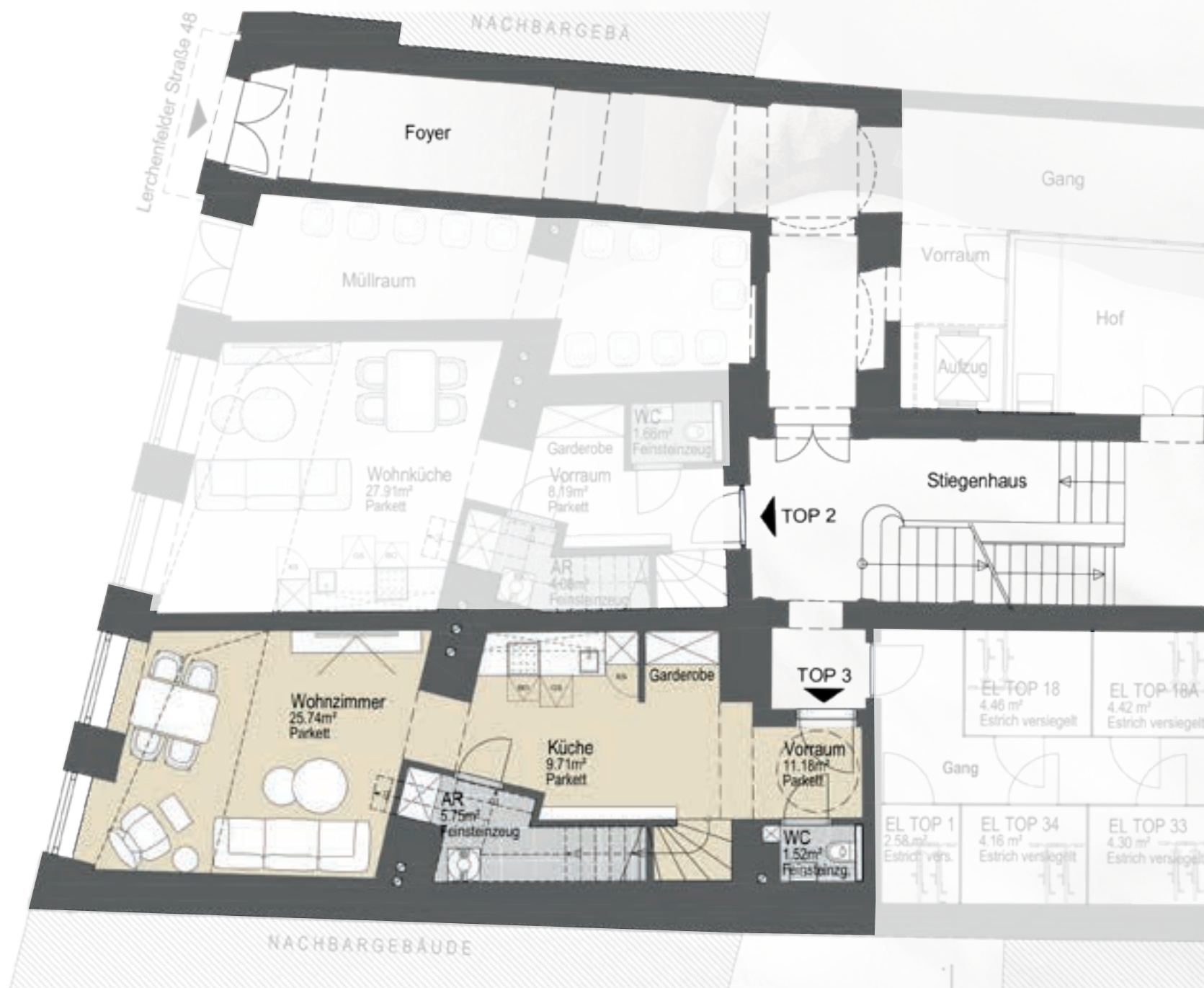
Erdgeschoß
