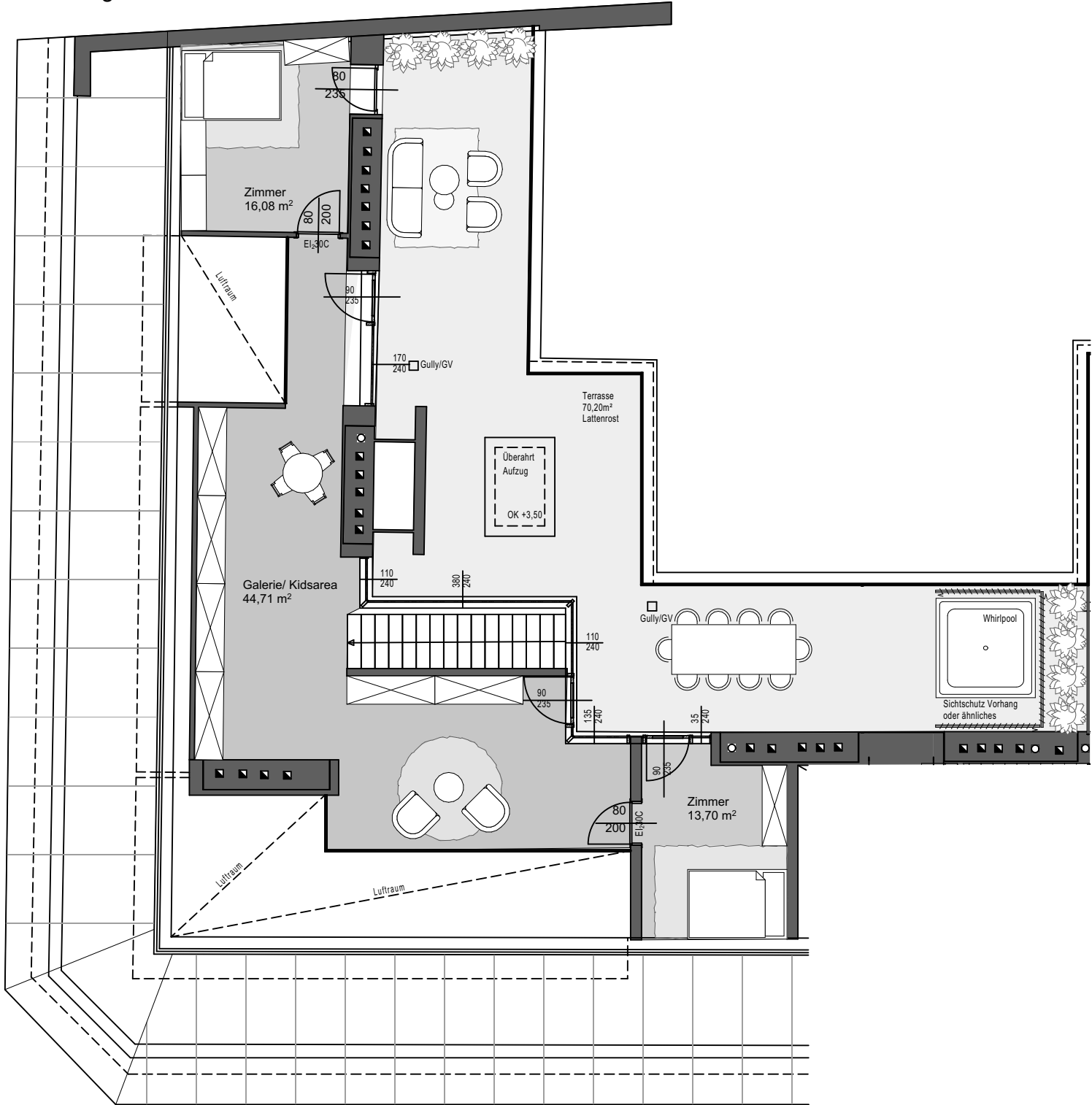
Terrassengeschoß
