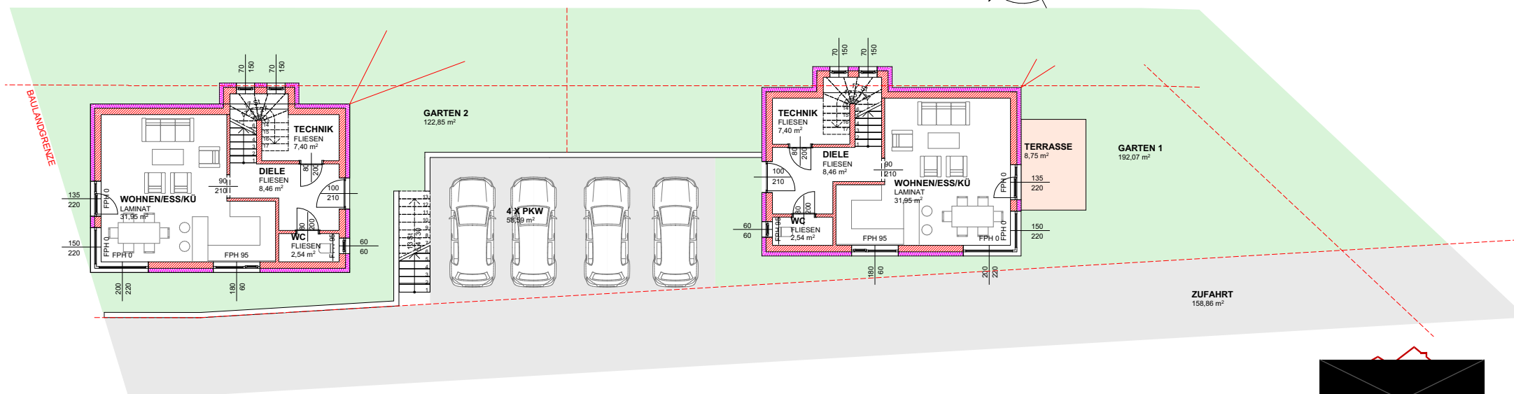
ERDGESCHOSS M:1:100
