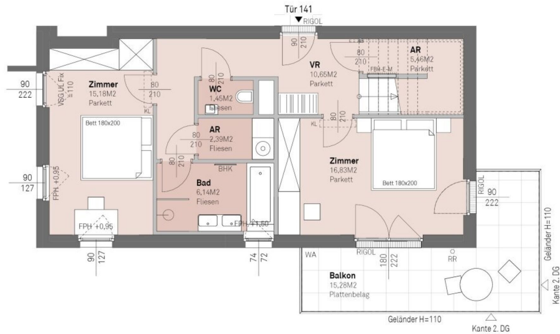
EBENE 1 - 1.DG
